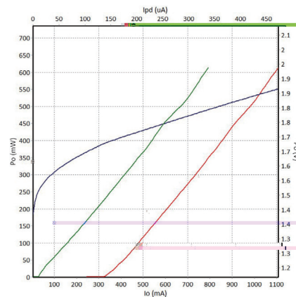
785nm P-I-V
